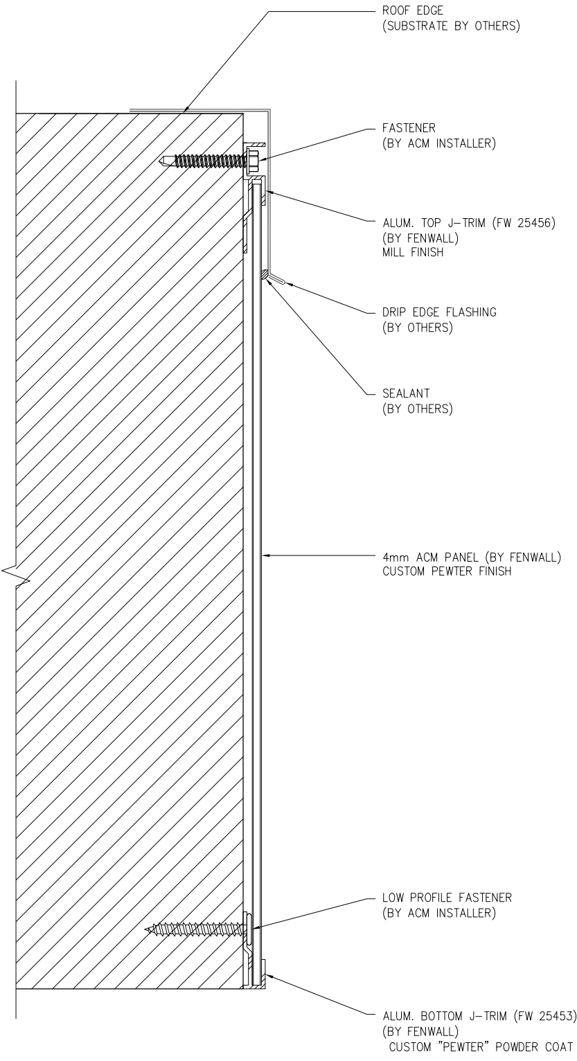
2 2 TOP J-TRIM (FW 25456) SECTION N.T.S.
