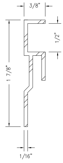
2 2 TOP J-TRIM (FW 25456) SECTION N.T.S.
