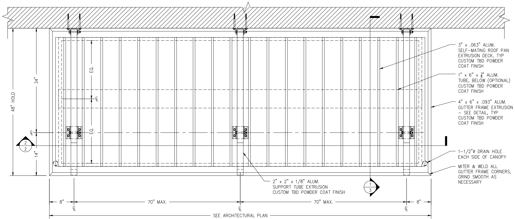
1 CANOPY 2 PLAN N.T.S.
