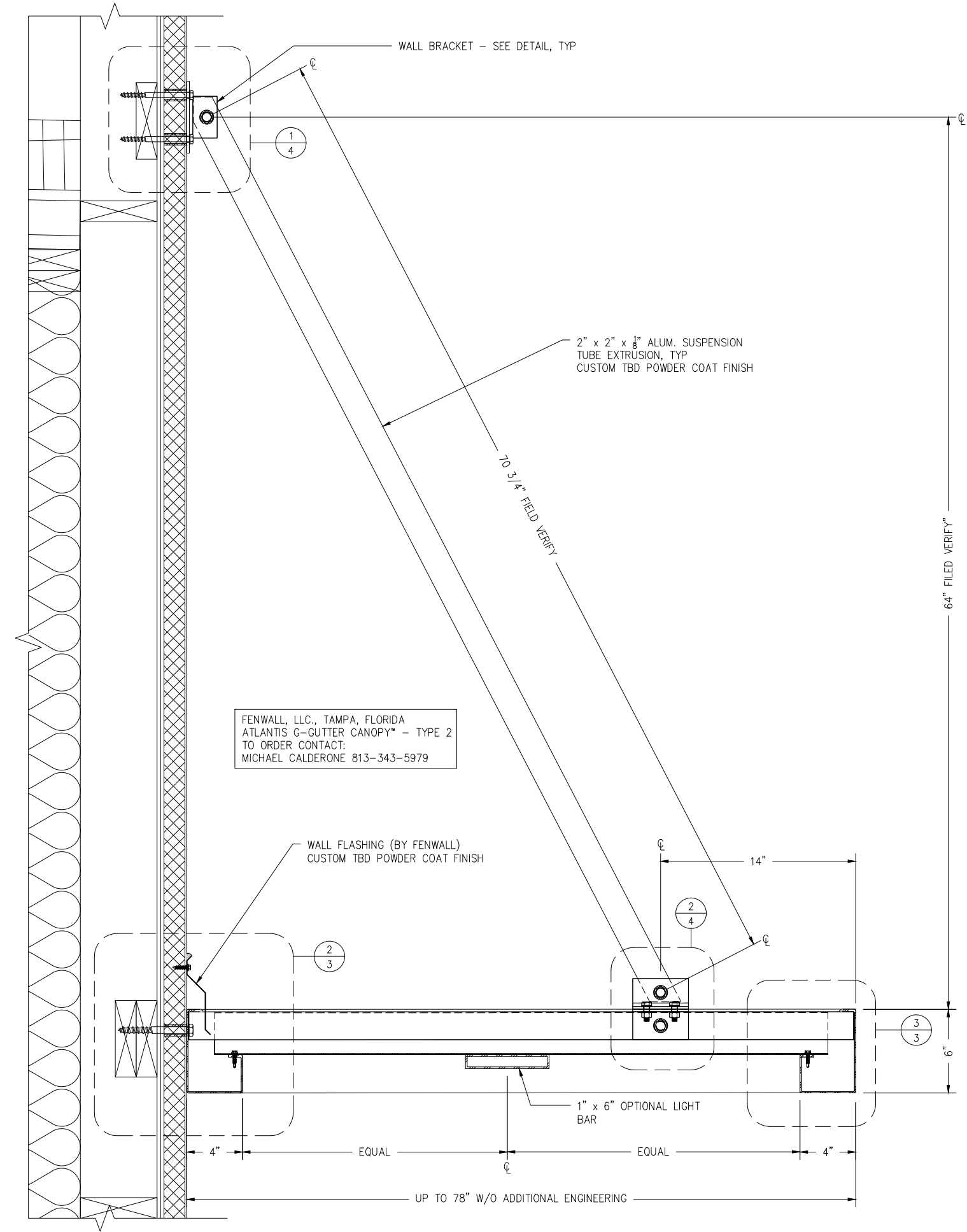
1 3 CANOPY TRANSVERSE SECTION N.T.S.
