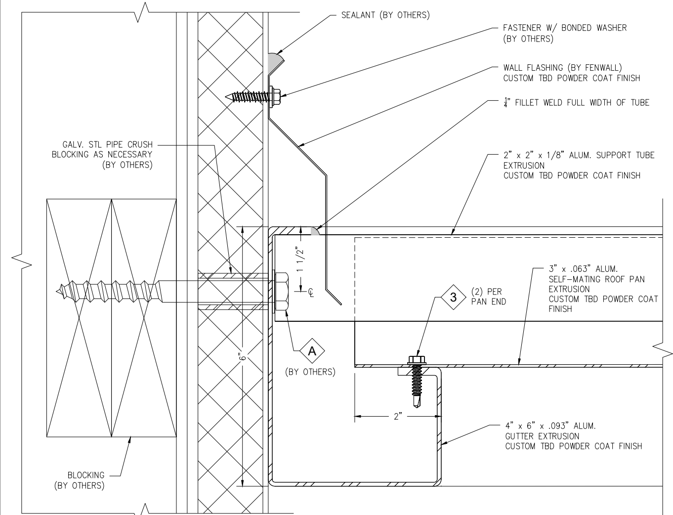
2 3 CANOPY DETAIL SECTION N.T.S.
