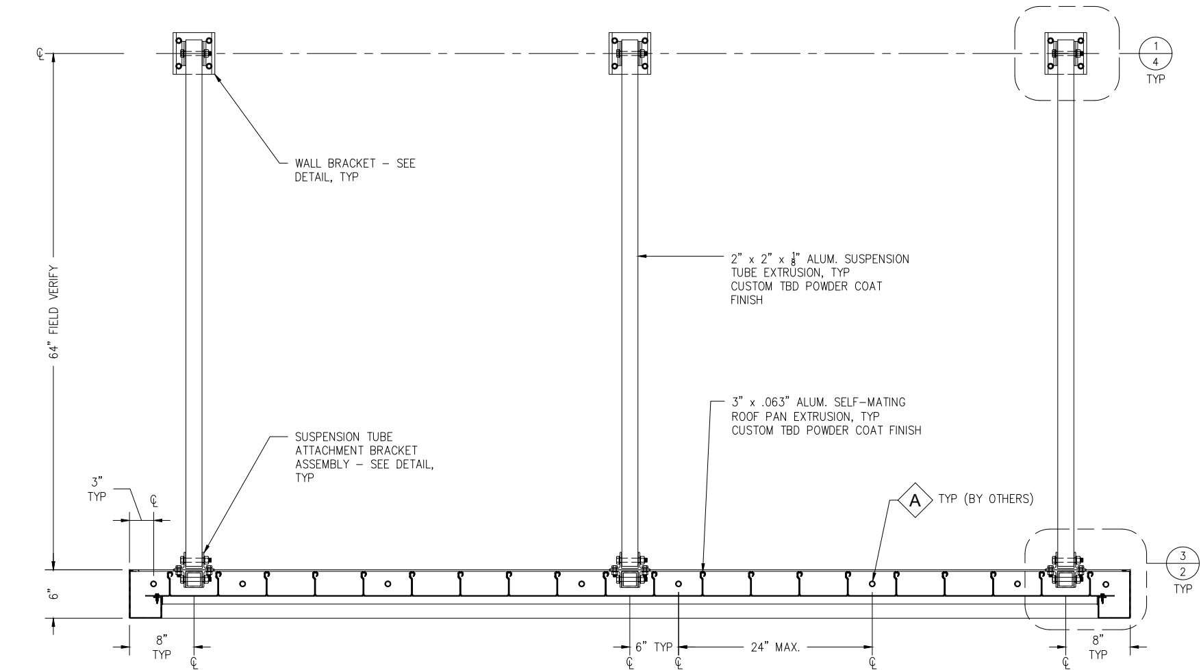
2 CANOPY 2 LONGITUDINAL SECTION N.T.S.
