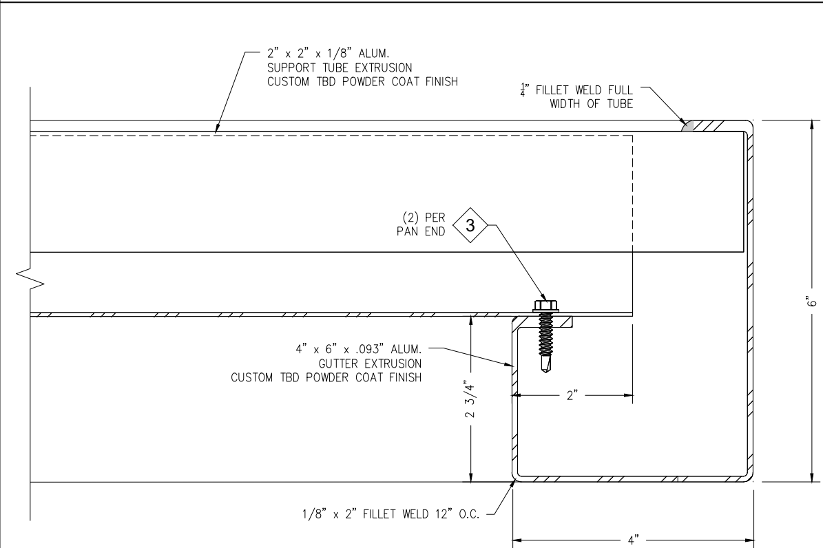
2 3 CANOPY DETAIL SECTION N.T.S.
