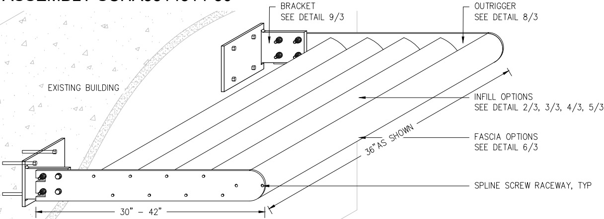
1 3 ECONO – SUNSHADE SIDE VIEW N.T.S.
