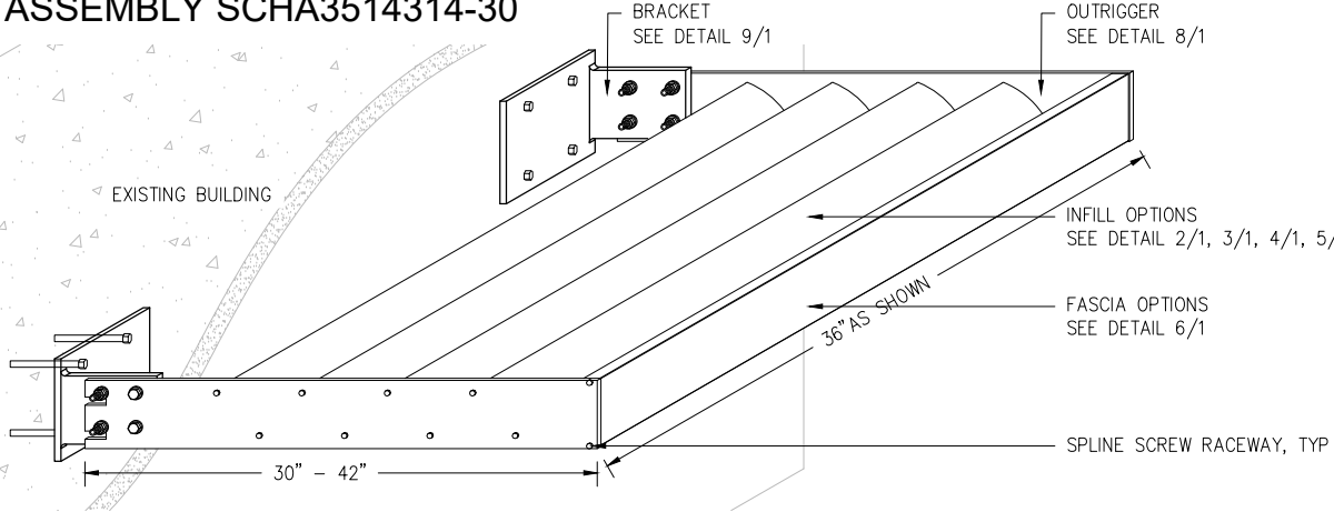
1 1 ECONO – SUNSHADE SIDE VIEW N.T.S.
