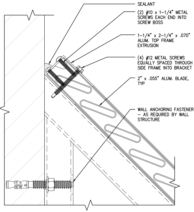
1 5 DETAIL ELEVATION N.T.S.
